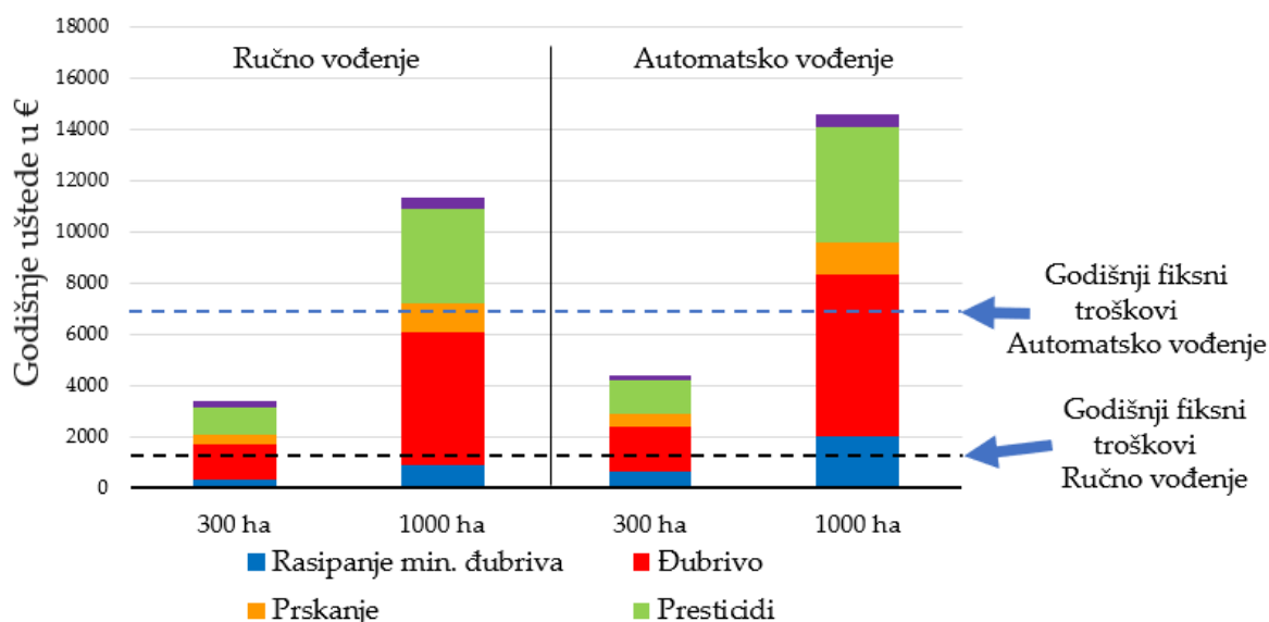
Slika 1.21. Grafikon prikazuje godišnje uštede u ratarskoj proizvodnji zbog primene GPS sistema navigacije kao posledicu smanjenja grešaka tokom uklapanja prohoda pri izvođenju različitih operacija. Troškovi uključuju i uštede u ljudskom i mašinskom radu (Reckleben, 2008).
